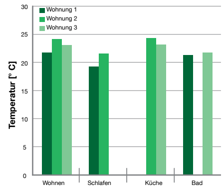
Abb. 83: Durchschnittliche Innenraumtemperaturen in den drei untersuchten Wohnungen
