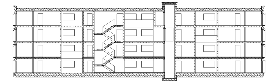
Abb. 132: Längsschnitt
