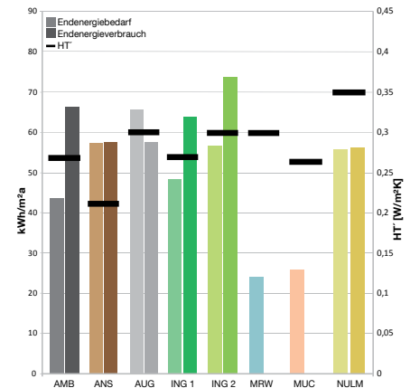
Abb. 153: Verhältnismäßigkeit der Transmissionswärmeverluste zu Endenergiebedarf bzw. -verbrauch
