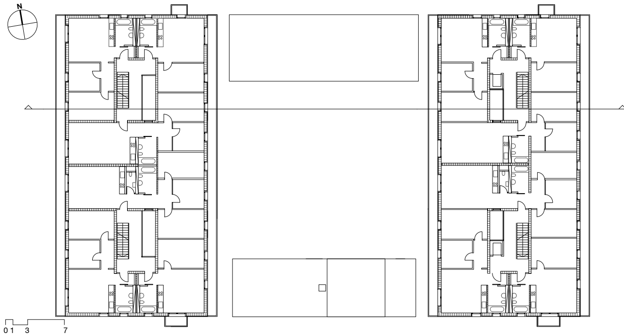
Abb. 47: Regelgrundriss 1. OG
