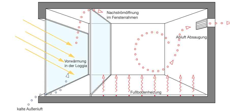
Abb. 163: Funktionsweise der passiven Solarnutzung durch Vorerwärmung der Luft in den Loggien
