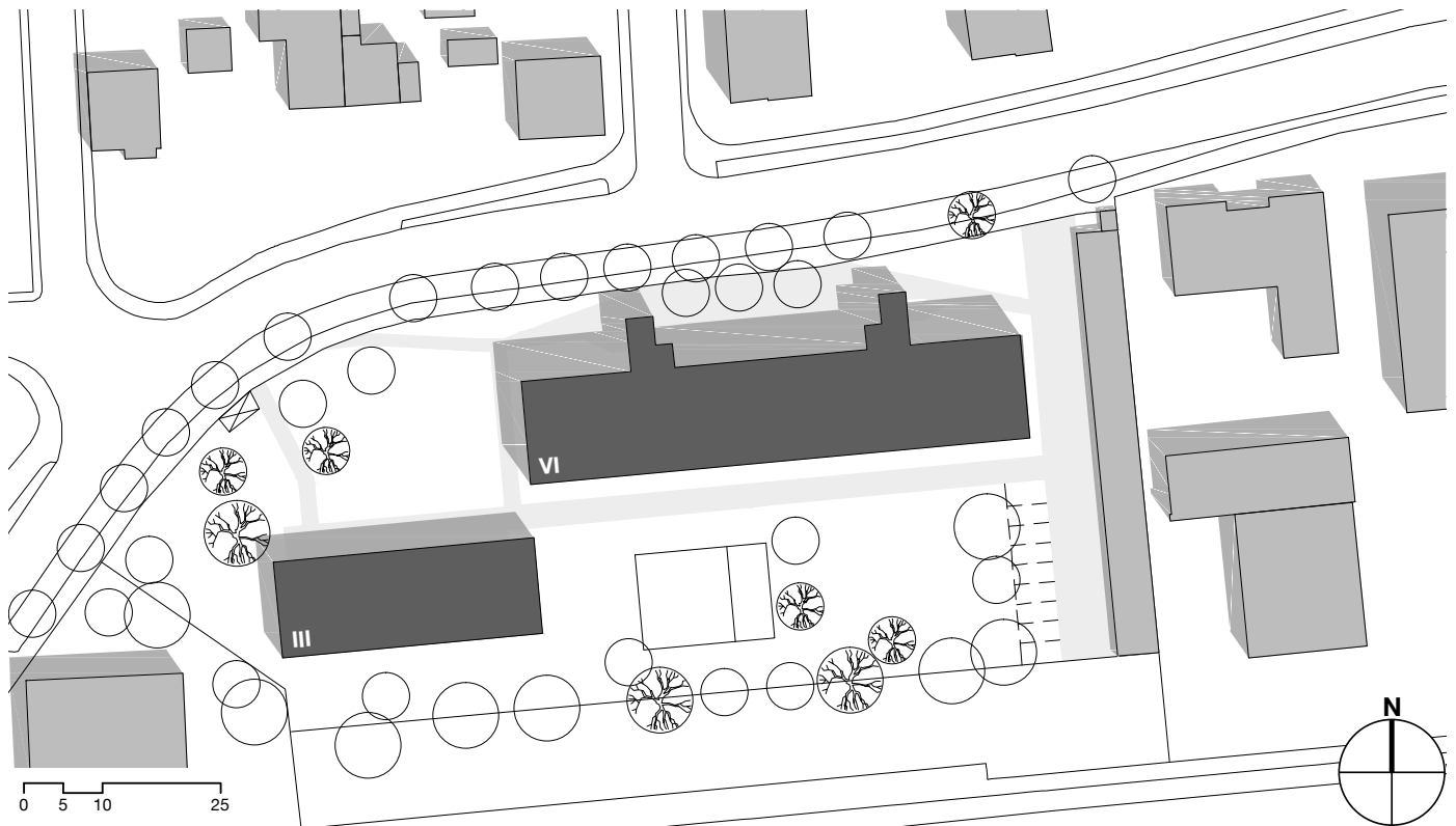
Abb. 28: Lageplan
