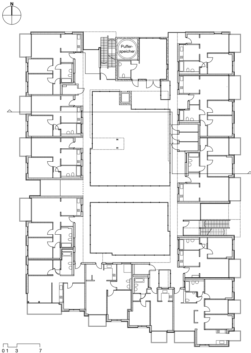
Abb. 86: Regelgrundriss 1.OG
