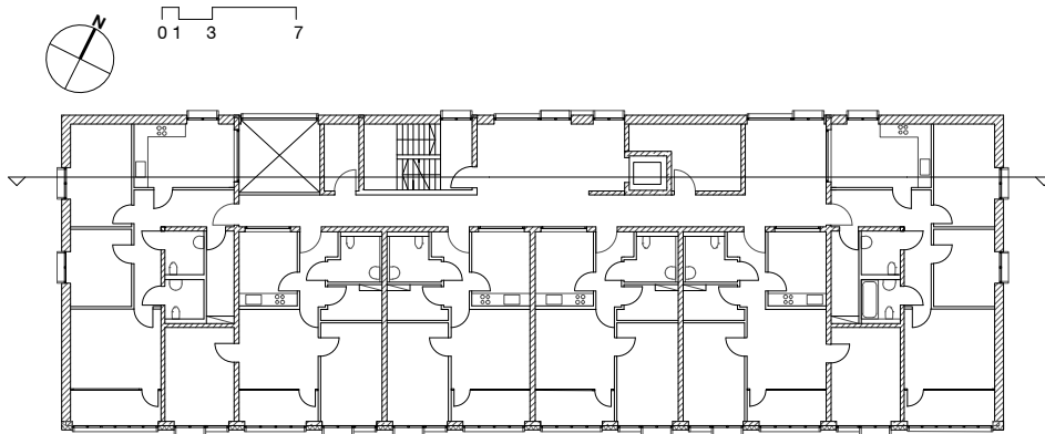
Abb. 130: Regelgrundriss 1.OG
