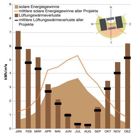
Abb. 53: Vergleich der solaren Energiegewinne mit den Lüftungswärmeverlusten
