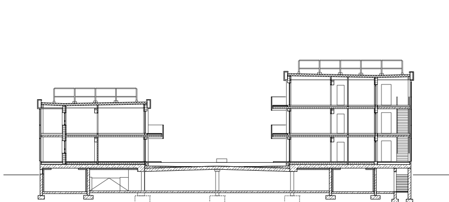
Abb. 69: Querschnitt durch zwei Baukörper
