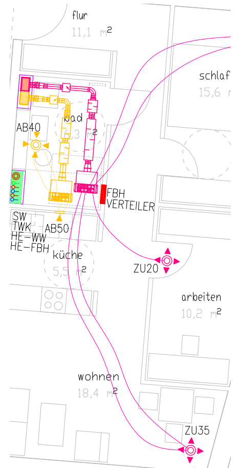
Abb. 126: Vertikale Leitungsverteilung in den Schächten und horizontale Verteilung der Lüftungsrohre in der Betondecke
