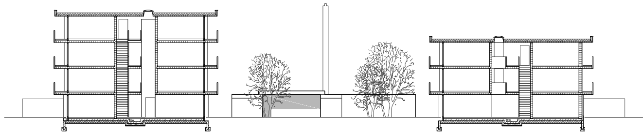
Abb. 48: Querschnitt
