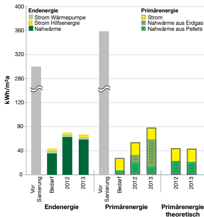
Abb. 25: Gegenüberstellung von Bedarf und Verbrauch
