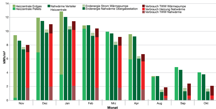
Abb. 24: Monatlicher Anteil der Wärmeherzeugungsort in der Heizzentrale sowie Verluste aus Erzeugung und Übergabe von November 2013 bis Oktober 2014
